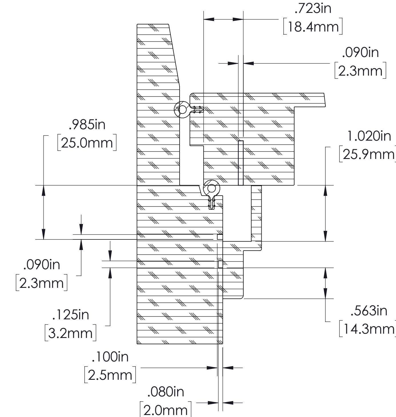
SECTION D-D SCALE 1 : 1
